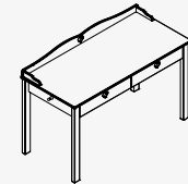
AMBU1314 W 1.300 mm - H 845 mm - D 600 mm
