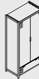
AXKL1219 W 1.000 mm - H 2.000 mm - D 550 mm
