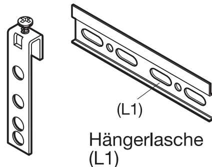
Halterung (vormontiert)
