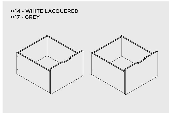
PILD90•• W 558 mm - H 396 mm - D 600 mm
