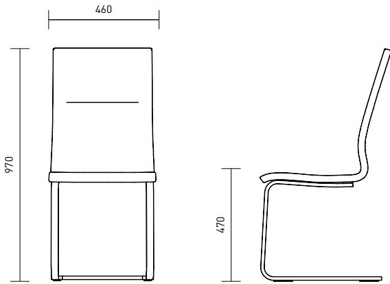
Freischwinger cantilever
